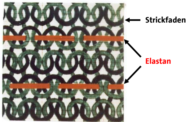
Abbildung 5: Maschenbild
